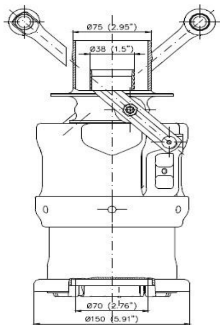
Accoupleur Mâle
